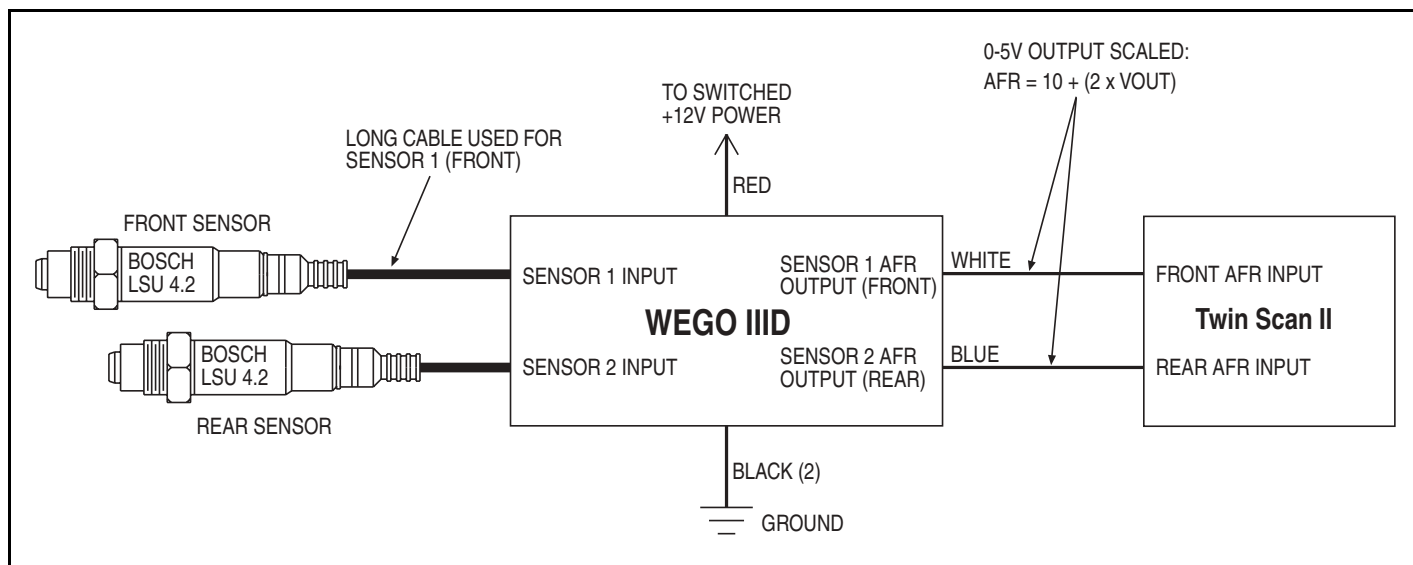
Figure 2 - WEGO Hookup
